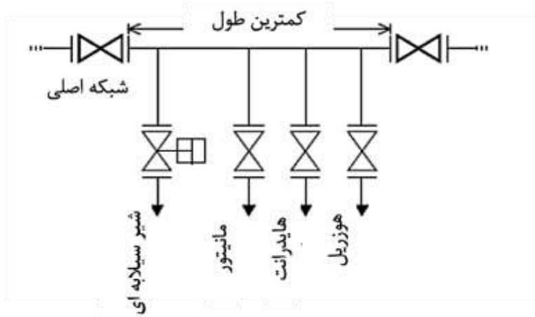
شکل ۳- نحوه انشعاب و اتصال به مصرف کنندگان آب آتش نشانی
